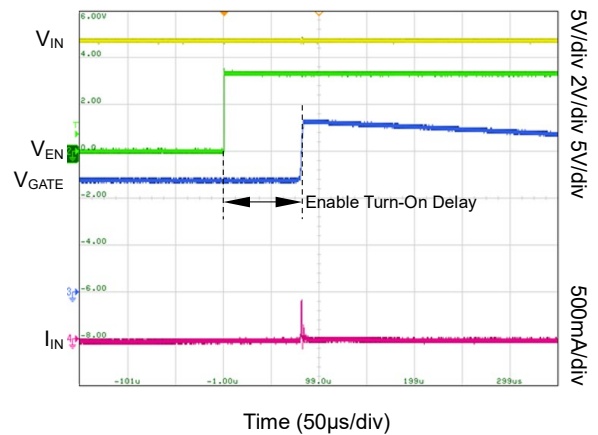
Enable Turn-On Delay
