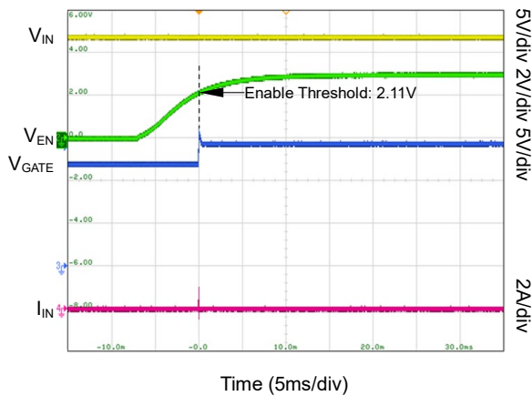
Enable Threshold
