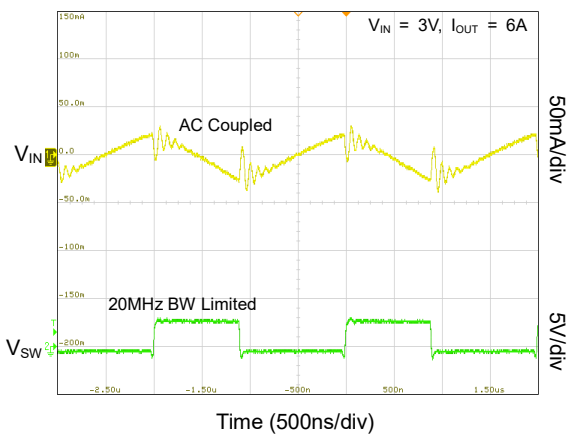
Input Ripple
