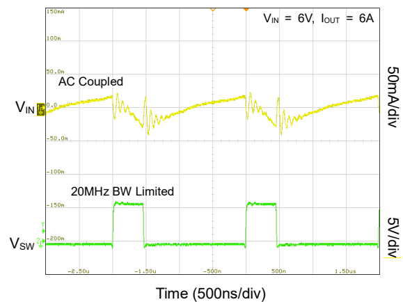
Input Ripple
