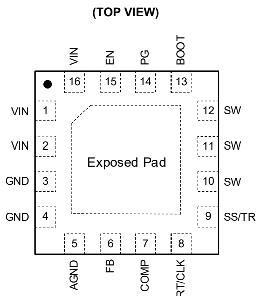
TQFN-3x3-16EL
