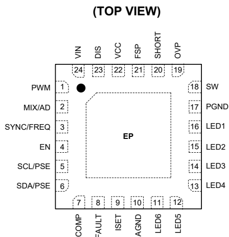
TQFN-4x4-24EL
