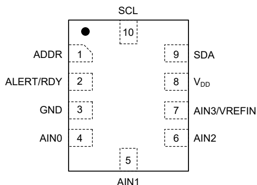
UTQFN-2x1.5-10L
