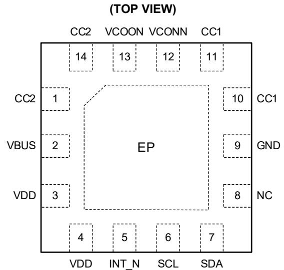
TQFN-2.5x2.5-14L
