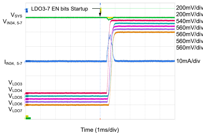
LDO3-7 EN bits Startup at I_{LDO3-7} = 0\text{mA}
