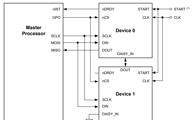
b). Daisy-Chain Configuration
