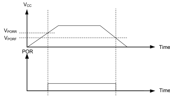
Figure 24. V POR
