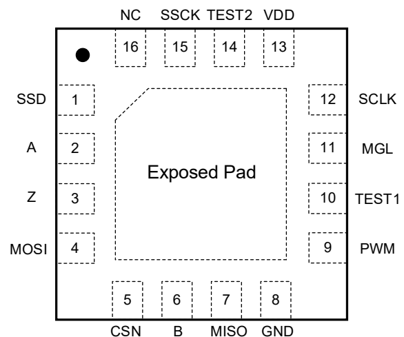
TQFN-3x3-16JL
