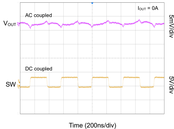
Output Ripple (SGMM2043B)
