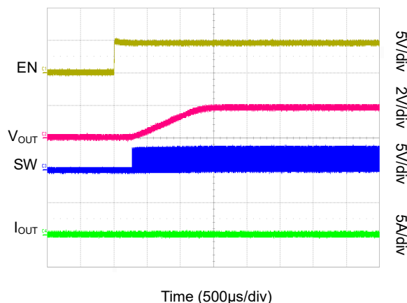
Startup without Load (SGMM2043B)
