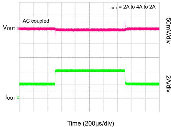
Load Transient (SGMM2043B)
