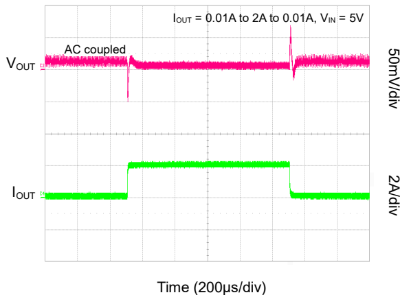
Load Transient (SGMM2043A)
