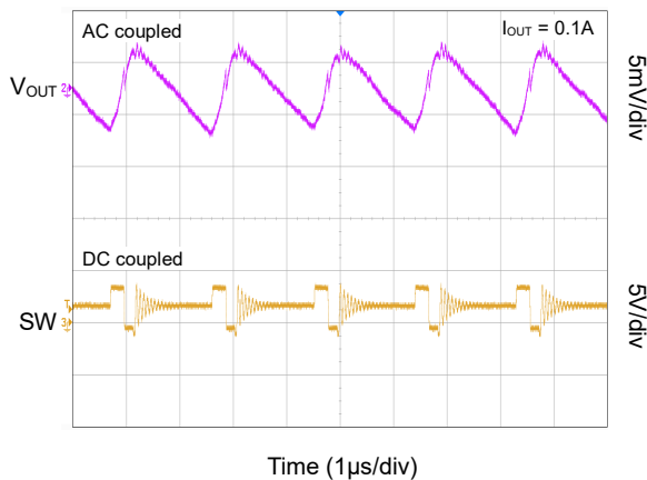
Output Ripple (SGMM2043A)
