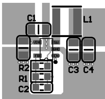
Top Layer
