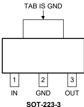
SGM2247xQ (TOP VIEW)
